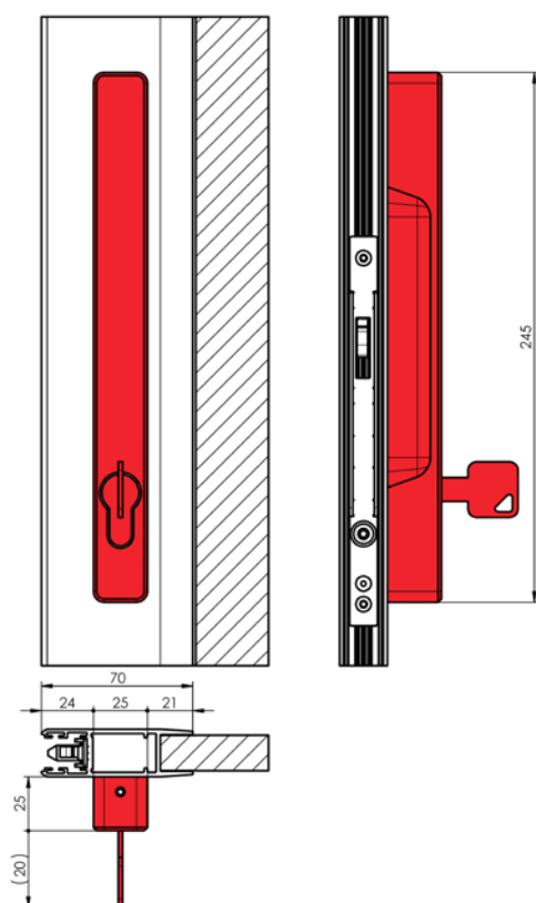
Uchwyt z zamkiem, zamykanie i otwieranie kluczem
