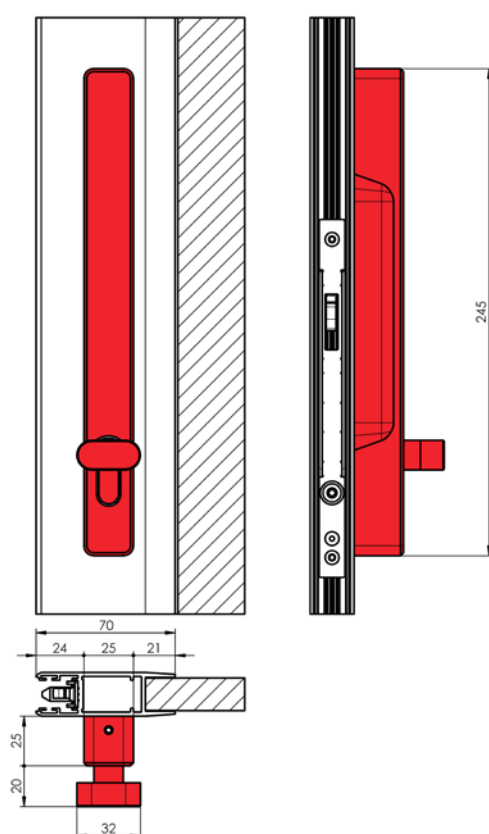
Uchwyt z zamkiem, zamykanie i otwieranie gałką
