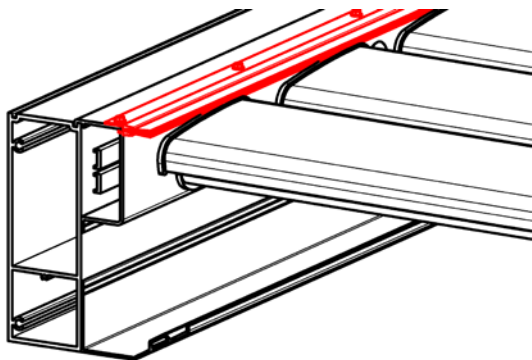
Szczotka uszczelniająca na stronę silnikową
