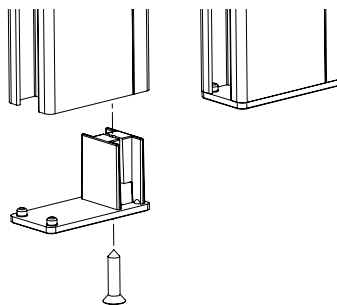
Ogranicznik końcowy na pomocniczej listwie prowadzącej
