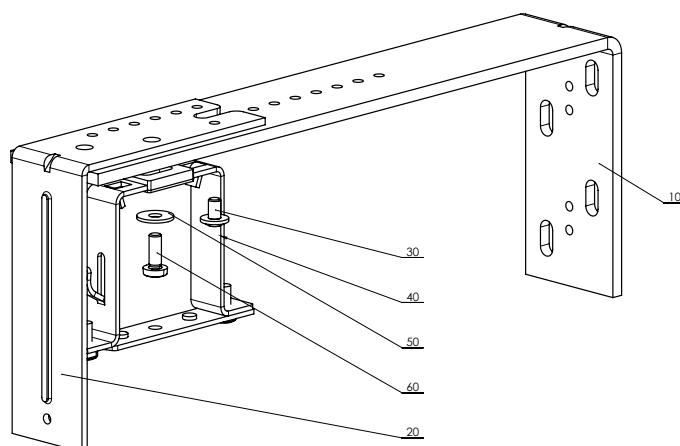
Uchwyt nastawny podwójny - stały 306 – 368 mm P 010/47 (2-01805-0000)
