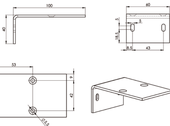
Listwa prowadząca GS 40 (7-303770-0000)
