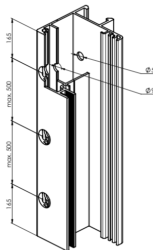
A849: wiercenie na przedniej stronie
