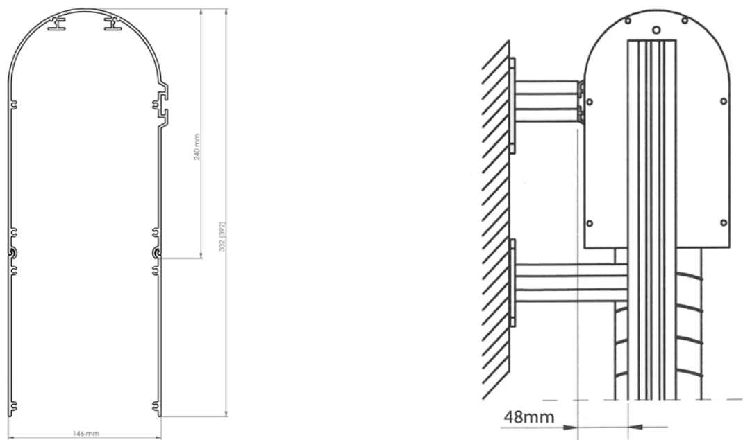
Przedłużenie kasety
