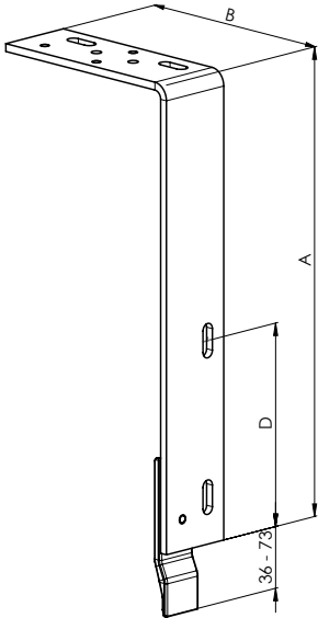
Uchwyt wariabilny P 130/5 2-01420-0000-0
