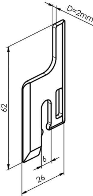
Podkładka dystansowa P 640 2-02670-XXXX-0
