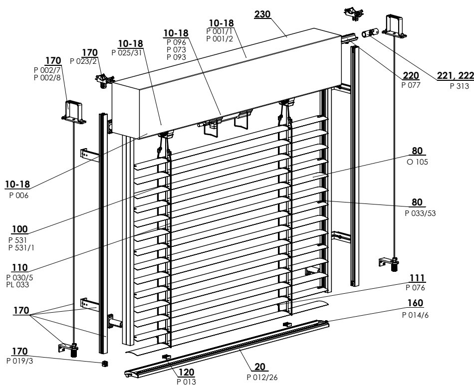
FLEXI 60 - MOTOR
