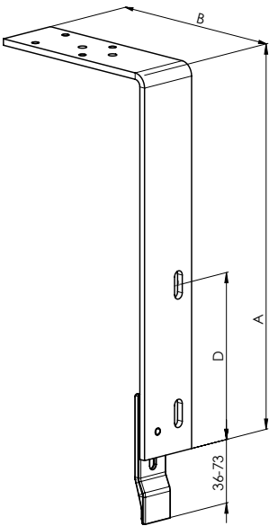
Uchwyt wariabilny P 130/4 2-01419-0000-0
