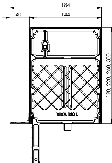
Przekrój kasety natynkowej VIVA + P 020/04, P 080/04, P 081/04 190x140b 220x140b 260x140b 300x140b
