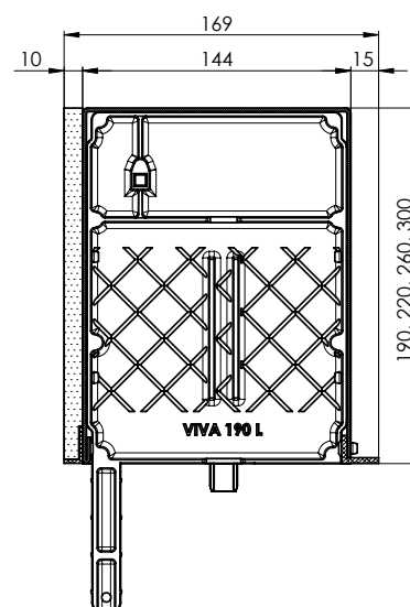
Przekrój kasety podtynkowej VIVA 190 x 169 x 2L x STY10 220 x 169 x 2L x STY10 260 x 169 x 2L x STY10 300 x 169 x 2L x STY10
