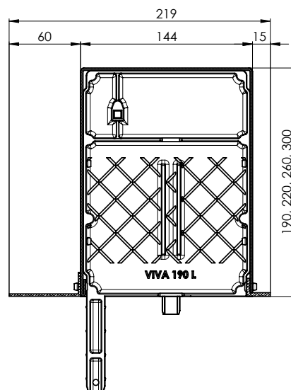
Przekrój kasety podtynkowej VIVA + P 020/06, P 080/06, P 081/06 190 x 150Lb 220 x 150Lb 260 x 150Lb 300 x 150Lb
