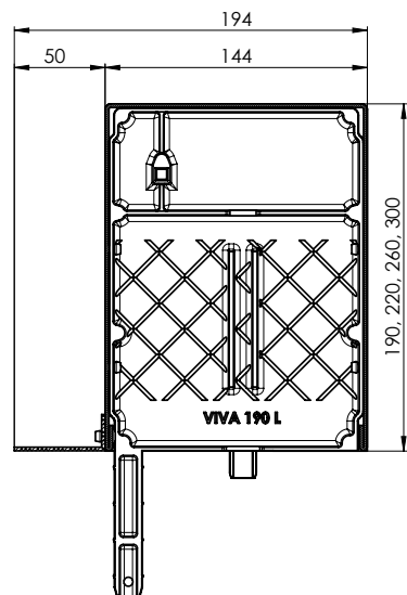
Przekrój kasety natynkowej VIVA + P 020/05, P 080/05, P 081/05 190 x 140b 220 x 140b 260 x 140b 300 x 140b
