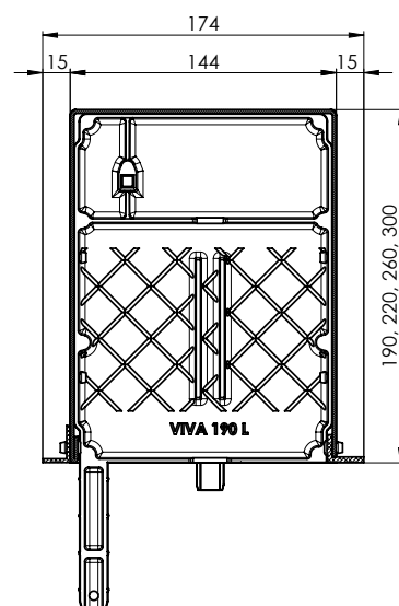
Przekrój kasety podtynkowej VIVA 190 x 160L2b 220 x 160L2b 260 x 160L2b 300 x 160L2b
