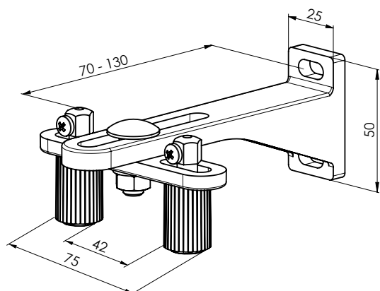
Prowadnica linki podwójna, 70 - 130 mm P032/8 (2-01652)
